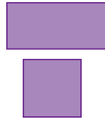
Rectángulos
