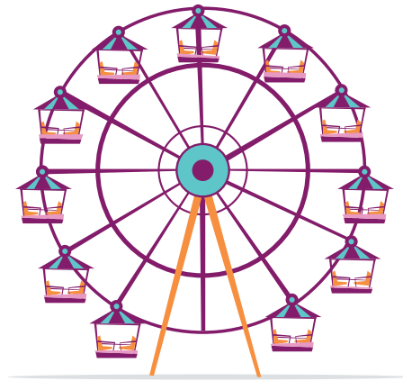
Movimiento circular
